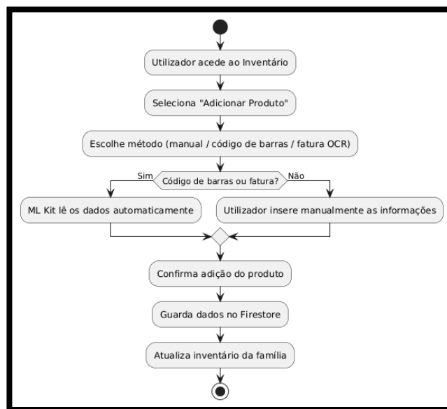
Figura 14 Diagrama de Atividade Adicionar Produto
