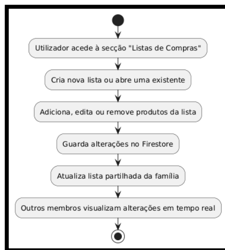
Figura 16 Diagrama de Atividade Gerir Listas de Compras
