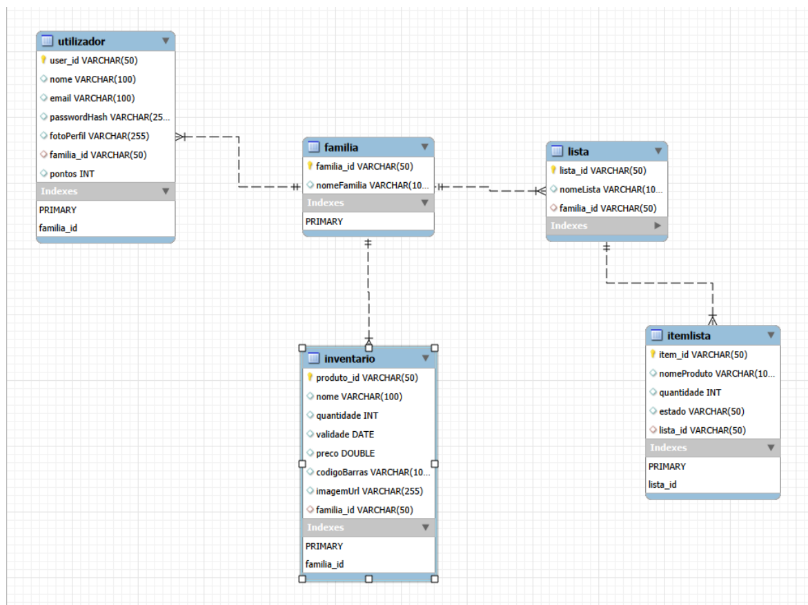
Figura 11 Diagrama Entidade-Relação
